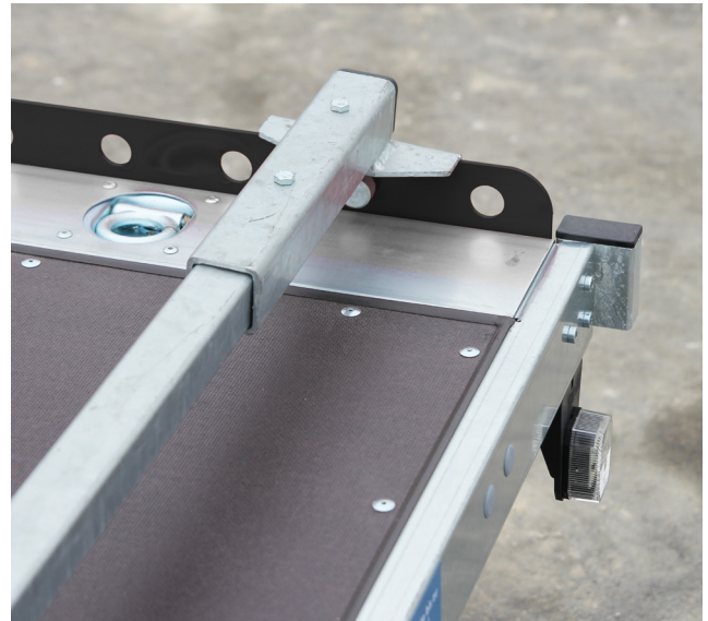
Radstopper (in Kombination mit Seitenschürze)
