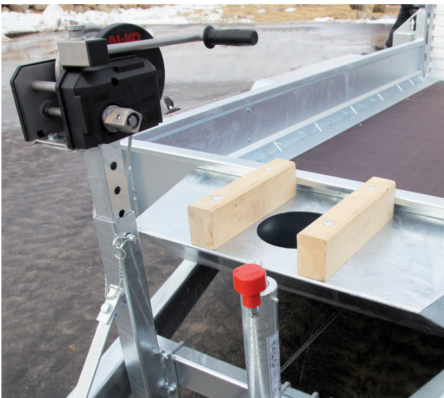
Baggerarmlaufe & Seilwindenbock inkl. Handseilwinde
