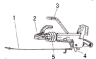
Bild 1: KNOTT Auflaufeinrichtung
