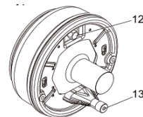
Schlüsselweite Nachstell-schraube (12)
